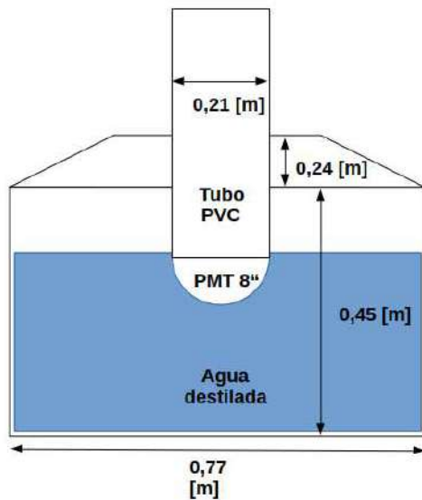
FIG. 3.— Esquema con las medidas del prototipo del detector Cherenkov de agua.
