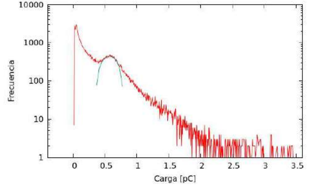
FIG. 16.— Histograma de cargas ajustado con una función f(x) = e^{a+bx+cx^2} , dando un valor para el VEM en el canal 0.57 \pm 0.06 pC con una energía de 90 MeV.
