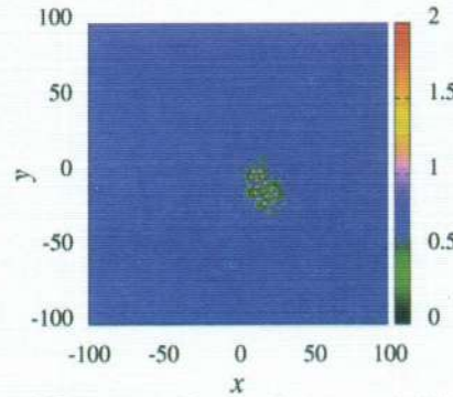
(d) Pentagon-grub, \gamma = 0.753 , \lambda_{\max} = 0.016 .
