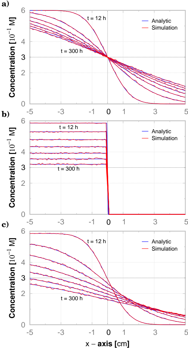
FIG. 7.— Resultados de una Ecuación de Fick (ver, Ec. (18)). Proceso: a) Difusión, b) Reacción y c) Difusión-Reacción.
