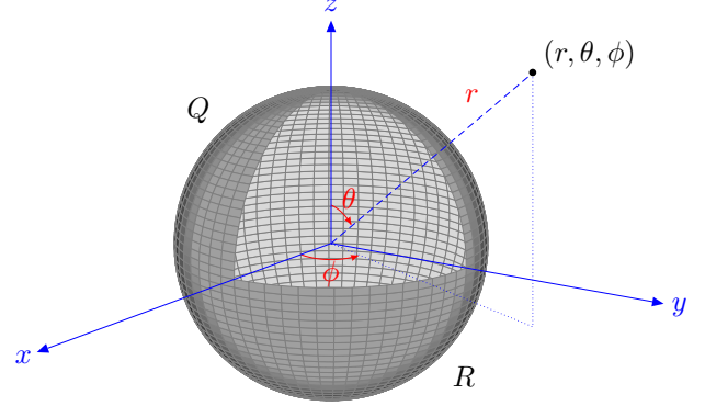
FIG. 3.— Representación esférica de un sistema de radio R con carga total Q presente en el espacio infinito.
